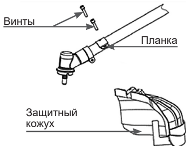
Рис. 3 Установка защитного кожуха
