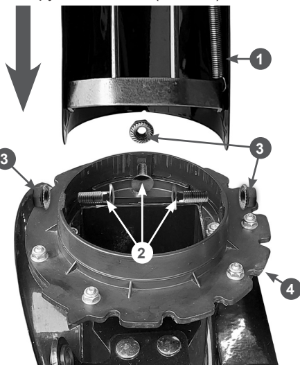
Рис. 14 Установка жёлоба выброса снега
