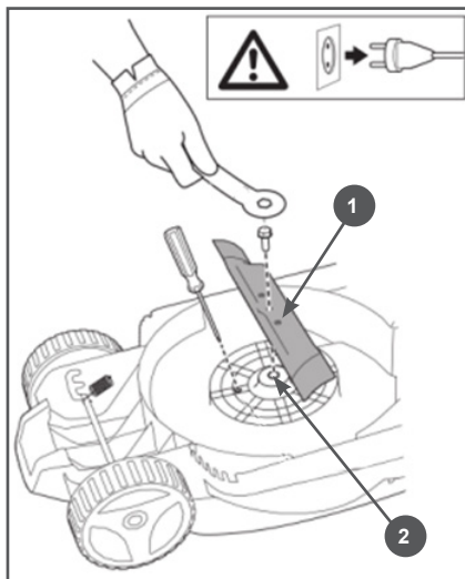
Рис. 10 Замена ножа
