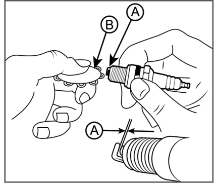
Рис. 13 Обслуживание свечи зажигания
