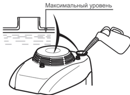
Рис. 7 Максимальный уровень топлива в топливном баке
