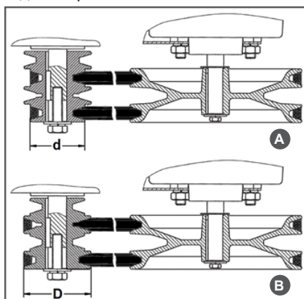
Рис. 26 Изменения передаточного числа ременной передачи
