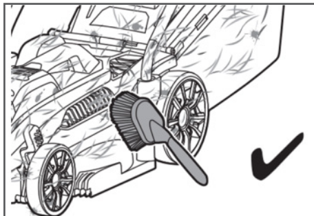
Рис. 14 Обслуживание вентиляционных отверстий охлаждения двигателя
