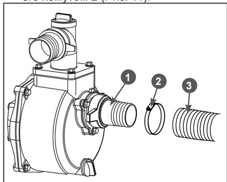
Рис. 11 Установка всасывающего рукава
