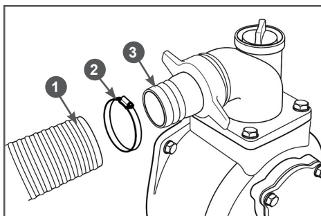
Рис. 14 Установка напорного рукава
