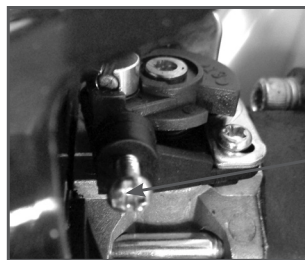
Рис. 16 Винт настройки оборотов холостого хода
