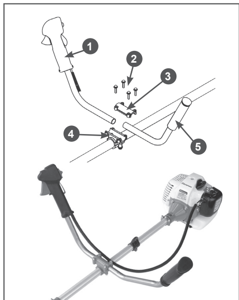
Рис. 4 Установка рабочей рукоятки
