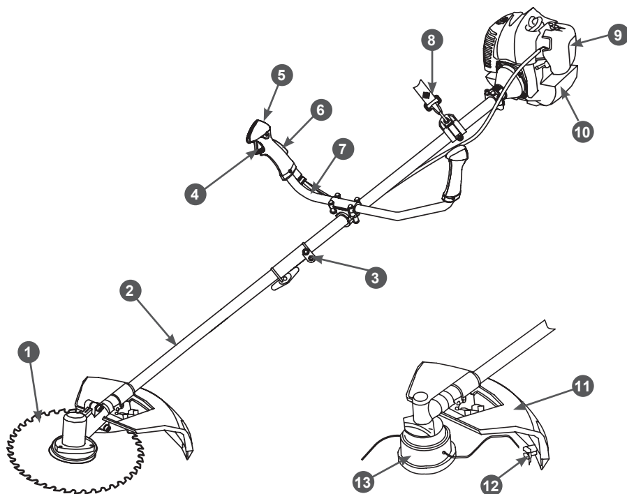
Рис.1 Расположение основных узлов и органов управления
