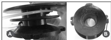
Рис.14 Установка корда
