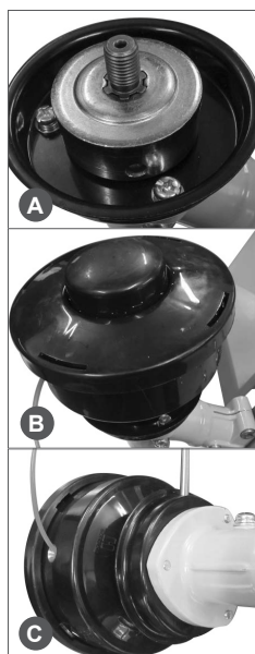
Рис. 6 Установка триммерной головк
