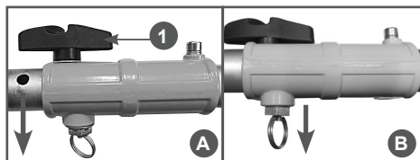
Рис. 3 Установка нижней части штанги
