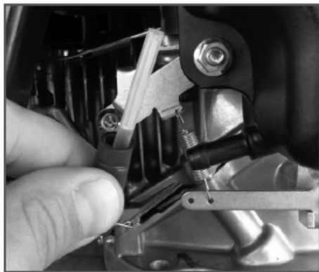
Рис. 16 Топливный фильтр
