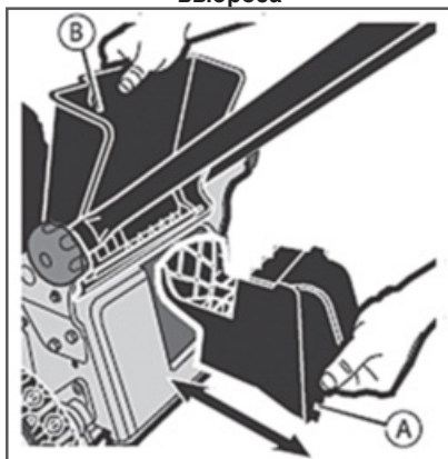
Рис. 4 Установка заглушки
