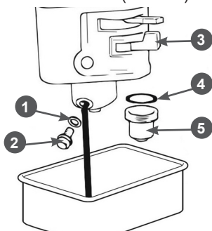
Рис. 24 Обслуживание карбюратора
