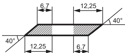
Размеры нового ножа
