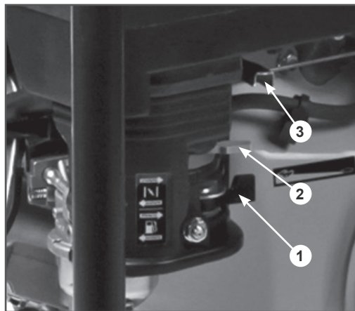
Рис. 4 Рычаги управления
