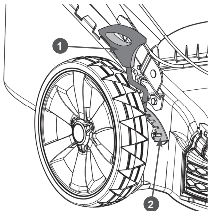
Рис. 13 Регулировка высоты скашивания
