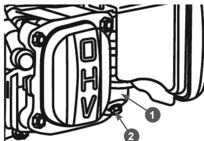
Рис. 21 Слив топлива из карбюратора
