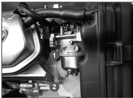
Рис. 27 Слив топлива из карбюратора
