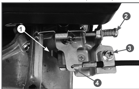
Рис. 10. Панель управления
