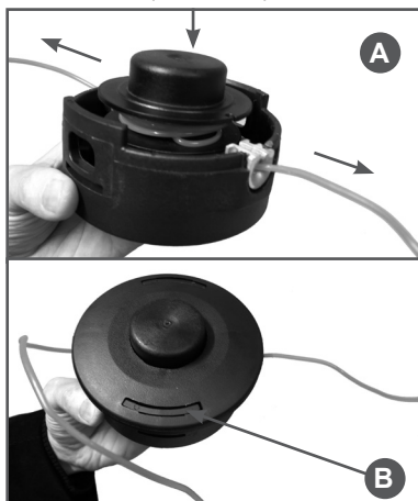
Рис. 19 Сборка триммерной головки
