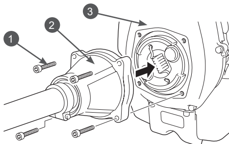
Рис. 5 Установка двигателя
