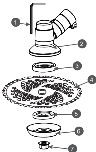
Рис. 3 Установка ножа
