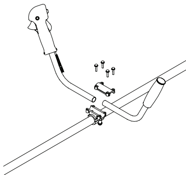
Рис. 6 Установка рукояток
