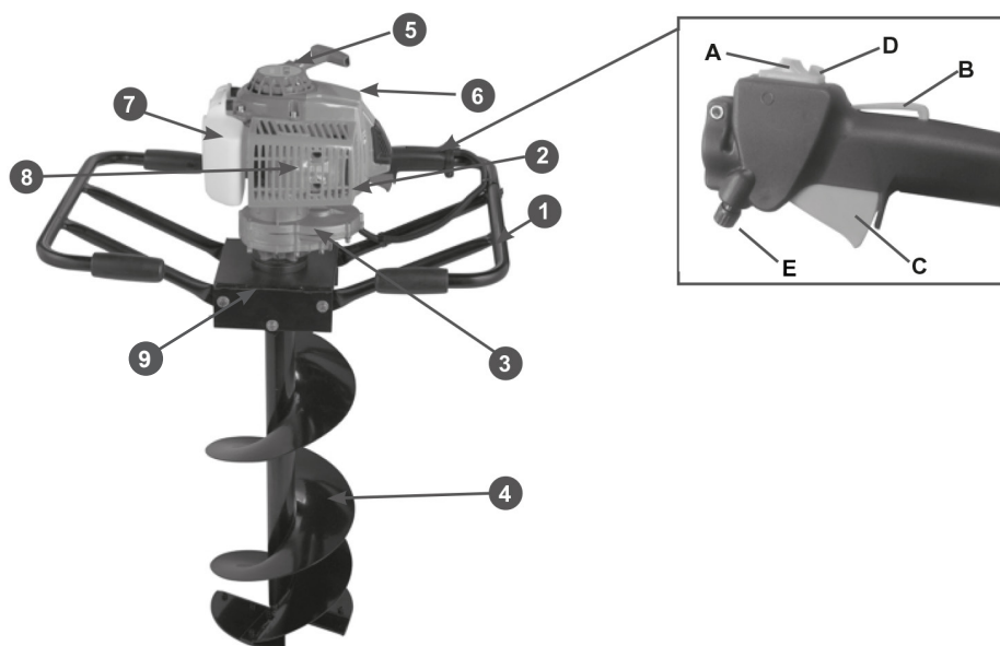
Рис. 1. Расположение основных узлов и органов управления мотобуrom
