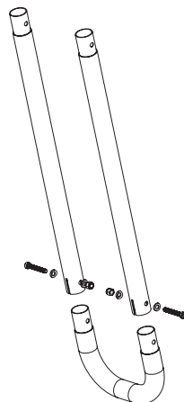
Рис. 3 Сборка задней опоры LSH5001H
