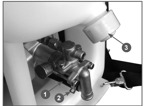
Рис. 8 Крышка сливного отверстия и шланг насоса
