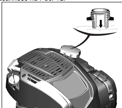
Рис. 12 Максимальный уровень топлива в топливном баке
