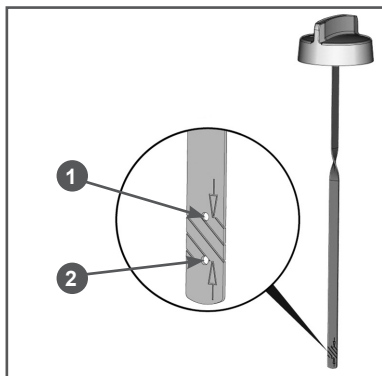
Рис. 20 Крышка-щуп маслосазливной горловины
