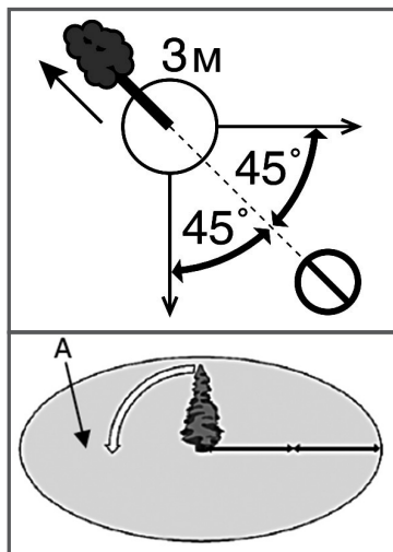
Рис. 10 Зона безопасности при валке дерева
