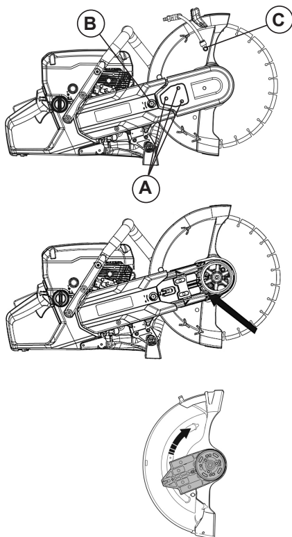
Рис. 7 Переустановка отрезного диска из центрального положения в положение снаружи
