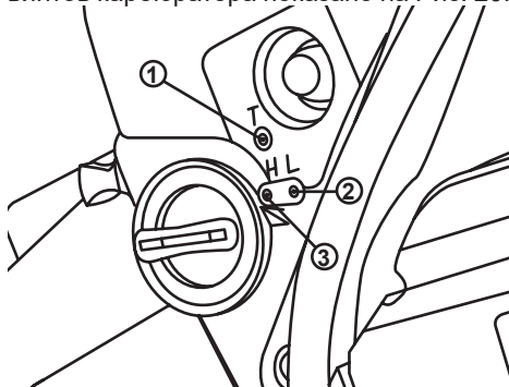
Рис. 20 Винты регулировки карбюратора 1 - винт «Т», 2 - винт «L», 3 - винт «H»
