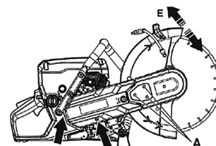
Рис. 25 Замена приводного ремня
