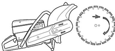
Рис. 5 Проверка направления вращения диска
