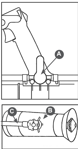
Рис. 19 Настройка дозатора
