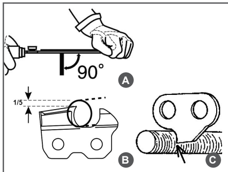
Рис.19 Заточка цепи
