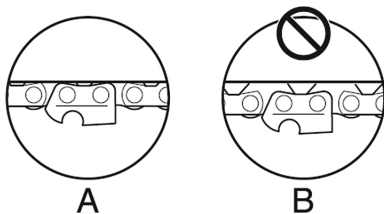
Рис. 4. Проверка натяжения цепи
