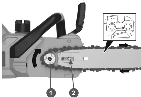
Рис. 3. Установка цепи
