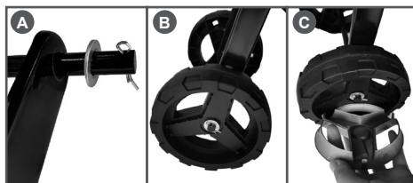
Рис. 2 Установка колес
