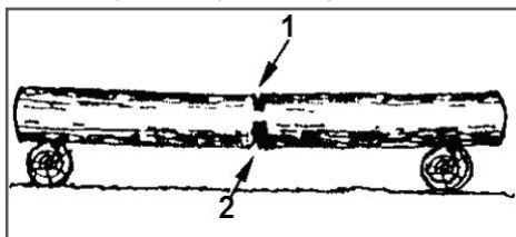
Рис. 15 Пропилы при раскрыжевке дерева на двух опорах
