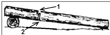
Рис. 16 Пропилы при раскрывке дерева на одной опоре
