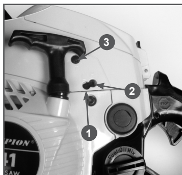
Рис. 20 Винты регулировки карбюратора
