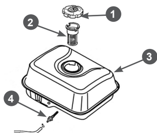
Рис. 21 Топливные фильтры
