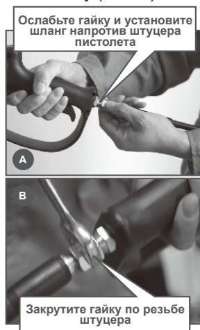
Рис. 3 Присоединение шланга высокого давления к пистолету
