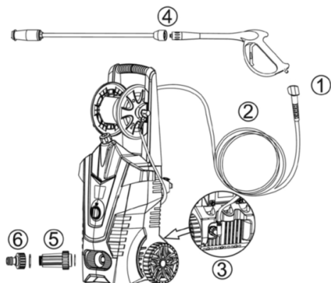
Рис. 2 Сборка аппарата
