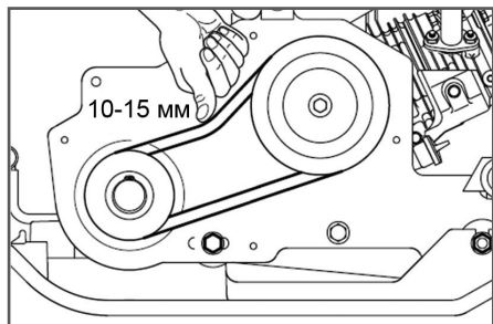
Рис. 24 Проверка натяжения ремня привода вибратора
