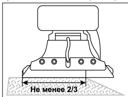
Рис. 14 Расположение виброплиты на краю обрабатываемой поверхности
