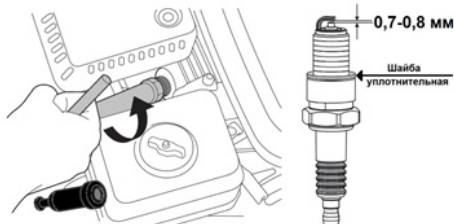
Рис. 19 Обслуживание свечи зажигания
