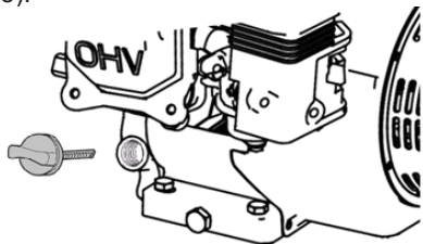
Рис. 5 Крышка-щуп маслосазливной горловины
