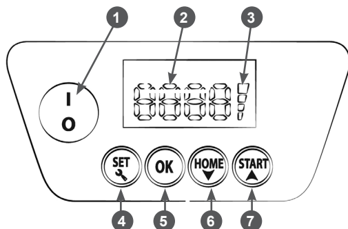
Рис. 3 Панель управления газонокосилки
