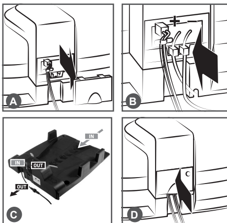
Рис. 11 Подсоединение ограничительного провода к зарядной станции
