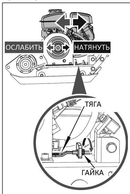
Рис. 30 Регулировка натяжения ремня PC5332F
