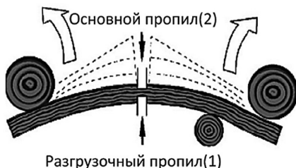
Рис. 13 Распиливание дерева, когда оба конца дерева зажаты и находятся под напряжением
