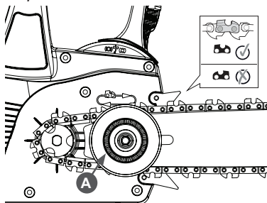
Рис. 3 Установка шины
