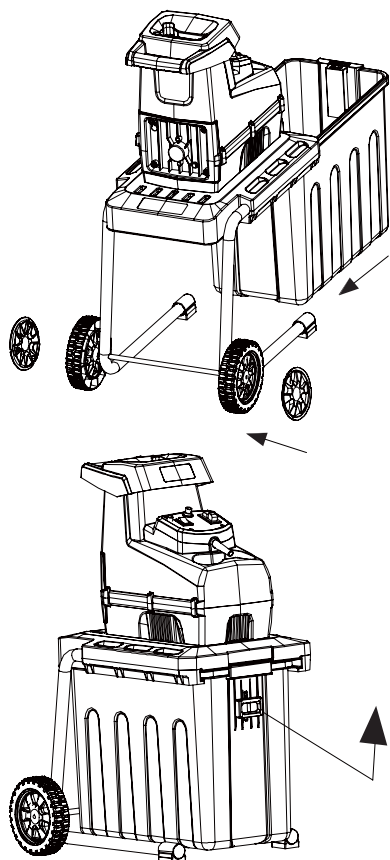
Рис. 4 Установка контейнера
