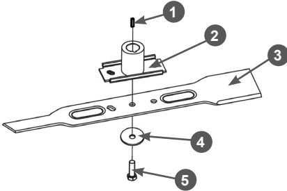
Рис. 23 Установка ножа
