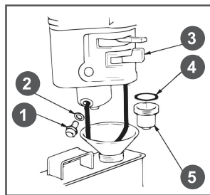
Рис. 20 Обслуживание фильтра-отстойника
