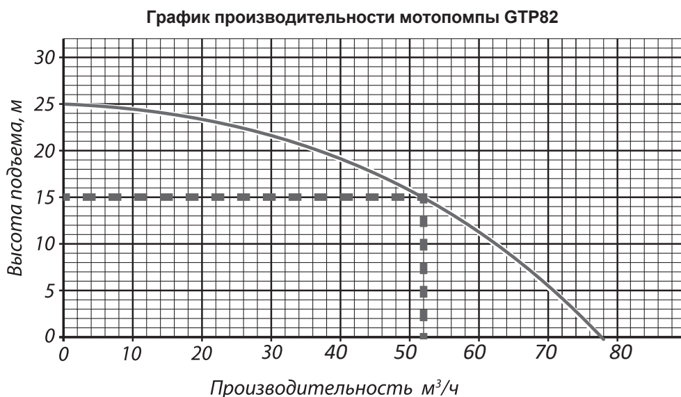
Рис. 24 График зависимости производительности мотопомпы от высоты подъема
