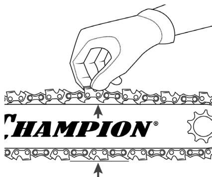
Рис. 5 Проверка натяжения цепи
