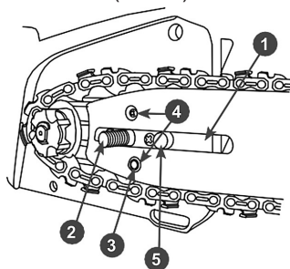
Рис. 4 Установка шины
