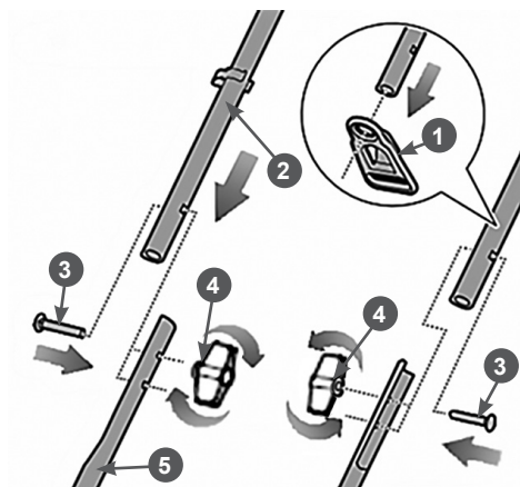
Рис. 4 Установка рабочей рукоятки
