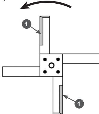
Рис. 4 Правильная установка фрез
