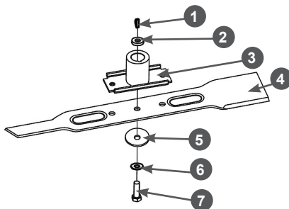
Рис. 24 Установка ножа
