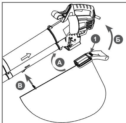
Рис. 6 Установка мусоросборника
