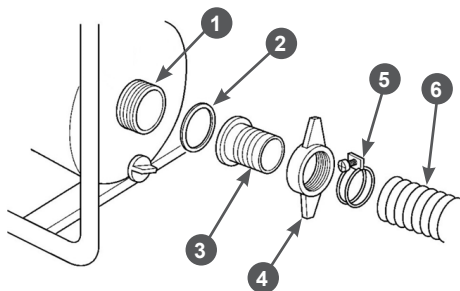
Рис. 11 Установка всасывающего рукава
