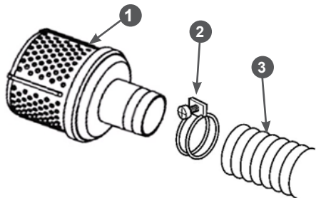
Рис. 10 Установка всасывающего фильтра
