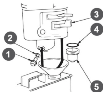
Рис. 21 Обслуживание фильтра-отстойника
