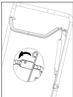
Рис. 2 Установка рычага и троса привода шнека
