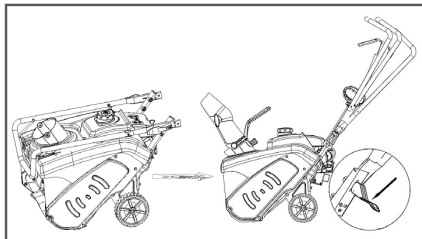
Рис. 3 Установка рабочей рукоятки Закрепите ручку стартера (Рис. 4).
