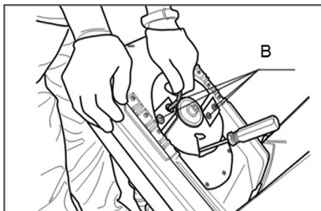
Рис. 9. Снятие ножей
