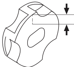
Рис. 23 Максимально допустимая глубина износа зубцов ведущей звездочки
