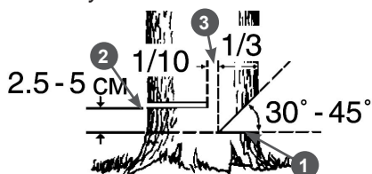
Рис. 10 Расположение запила, пропила и недопила
