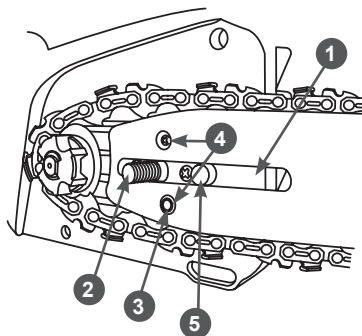
Рис. 4 Установка шины
