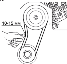
Рис. 23 Проверка натяжения ремня привода вибратора
