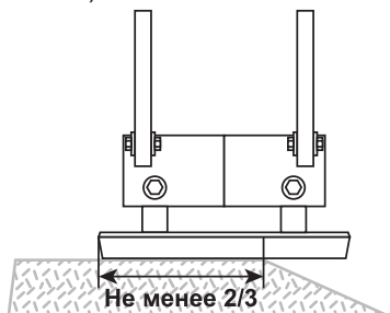
Рис. 12 Расположение виброплиты на краю обрабатываемой поверхности
