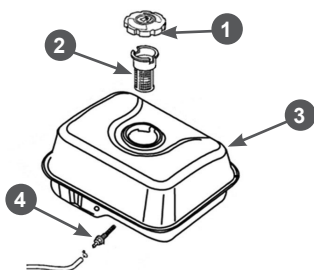
Рис. 16 Топливные фильтры
