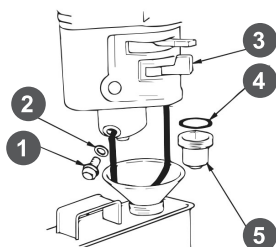
Рис. 18 Обслуживание фильтра-отстойника
