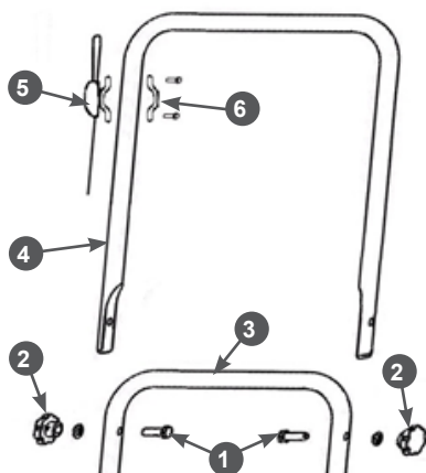
Рис. 2 Установка рабочей рукоятки
