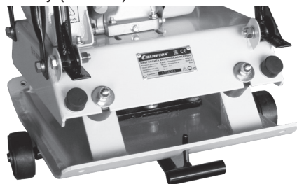
Рис. 25 Использование транспортировочной тележки
