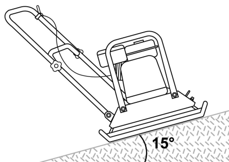
Рис. 13 Максимальный угол наклона виброплиты
