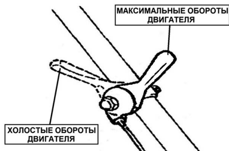
Рис. 10 Рычаг газа
