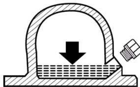
Рис. 22 Уровень масла в вибраторе
