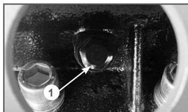
Рис. 21 Пробка контрольного отверстия 1. Пробка контрольного отверстия
