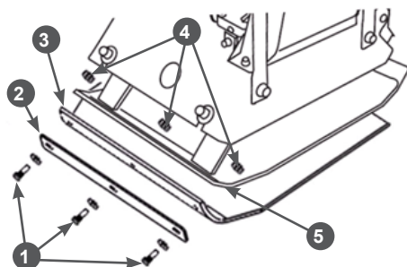
Рис. 3 Установка резинового коврика
