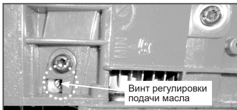
Рис. 11 Расположение регулировочного винта подачи масла
