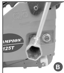
Рис. 4 Затяжка гайки крепления крышки шины
