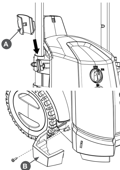
Рис. 2 Установка держателей для пистолета
