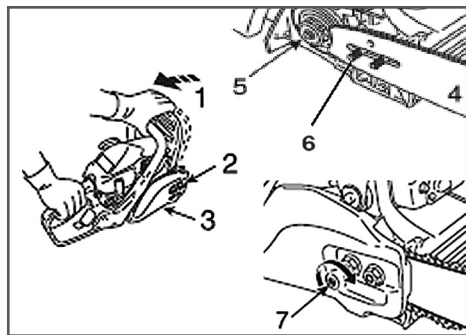
Рис. 2 Установка шины
