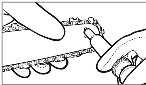
Рис. 26 Смазывание ведомой звездочки шины
