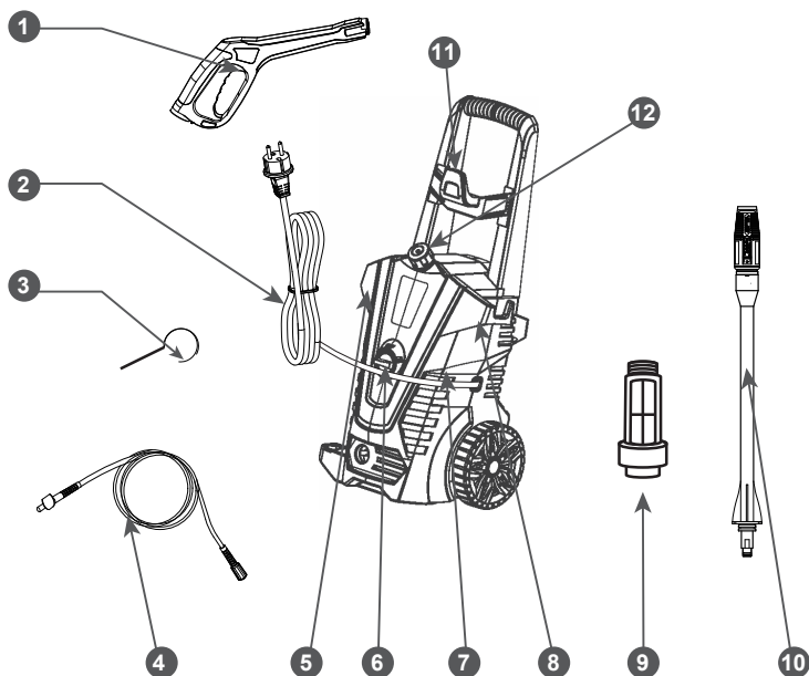
Рис. 1 Основные узлы и органы управления
