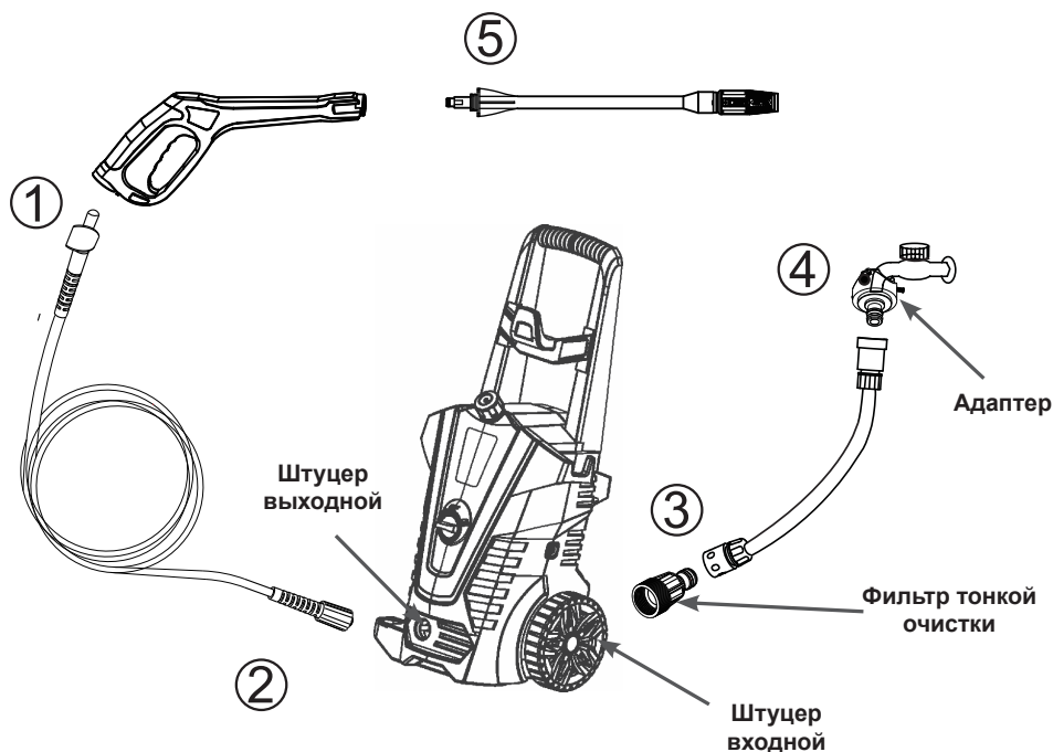
Рис. 2 Сборка аппарата
